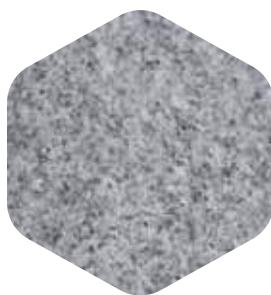
Цветок Урала
