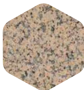
Жельтау 2
