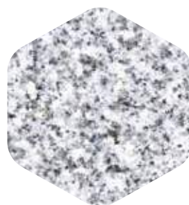
Санарское
