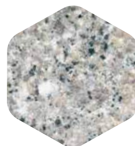
Капал-Арасан
