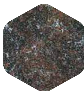
Гранатовый амфиболит
