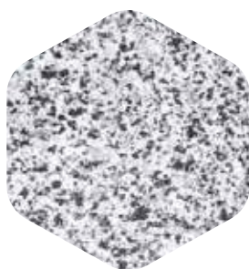
Покостовское
