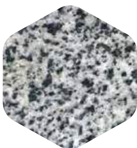
Камбулатовское
