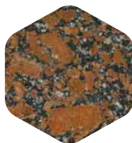
Капустинское
