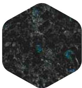
Волга Блю
