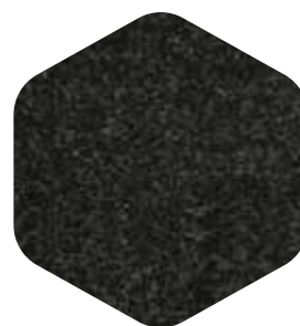
Габбро
